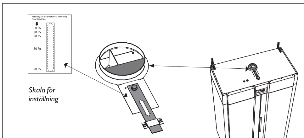
Spjäll för justering av tryckfallet i evakueringskanalen
