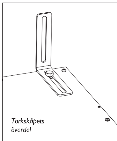
Vinkelkonsol för infästning i vägg
